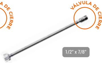
Tubo de abasto para inodoro 2120V26006000 40 cm, acero inoxidable con válvula reguladora.
